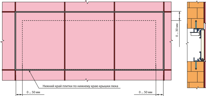
Примерная схема расположения облицовочной плитки
